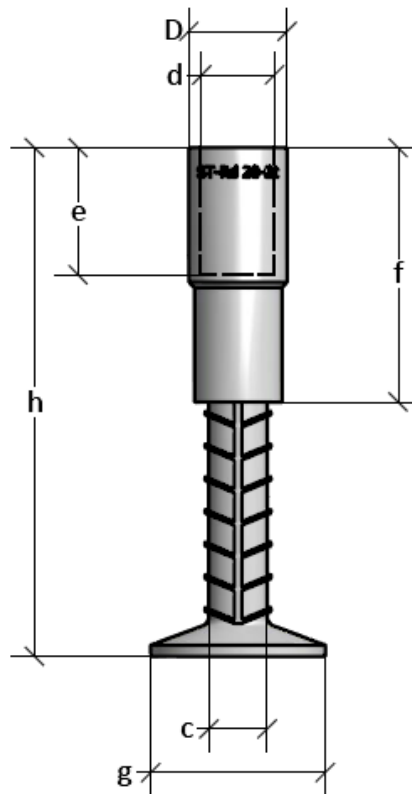
Kuva 2.1: Mittojen tunnukset.
