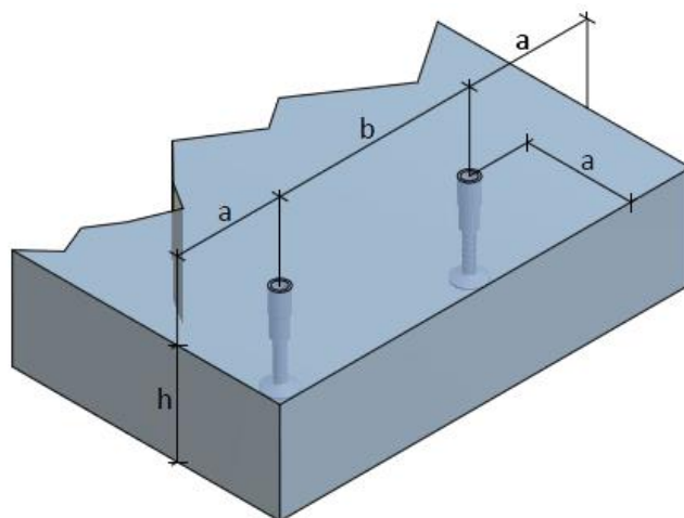
Kuva 6.1. Etäisyyksien tunnuksat
