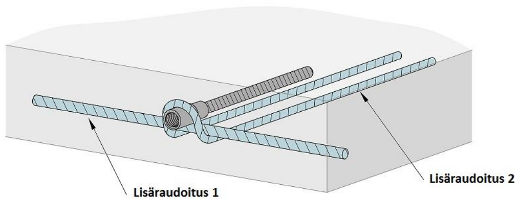
Kuva 5.2. Kyljestä noston lisäraudoitus
