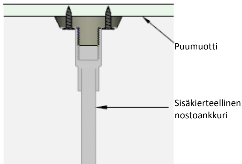
Kuva 7.1. Puumuotti ja nostoankkuri
