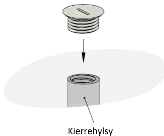
Kuva 7.2. Ankkurin kierrehylsy
