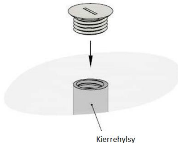
Kuva 7.9 Ankkurin suojaaminen ST-suojatulpalla
