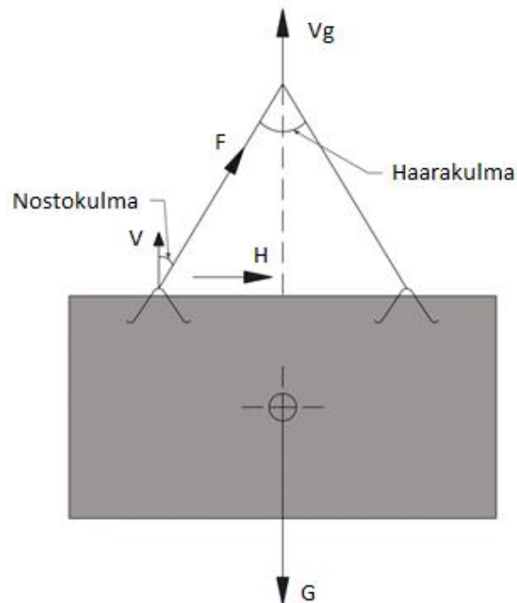
Kuva 5.1. Vino nosto
