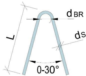
Kuva 6.2. Vinon noston lisäraudoitus
